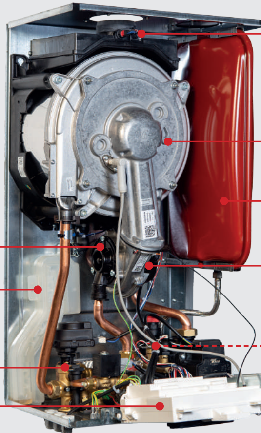
Doppia sonda sicurezza fumi
