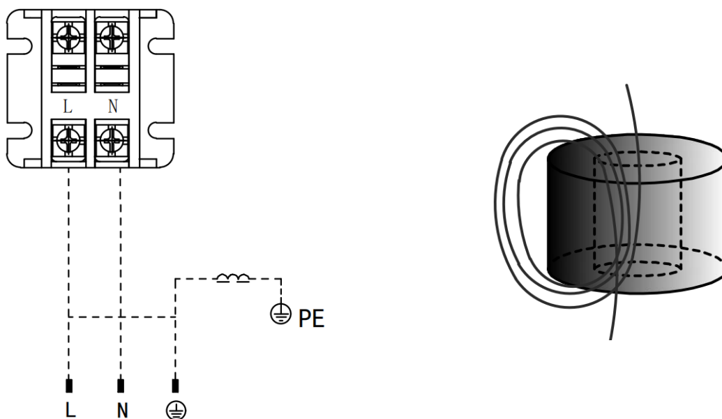
Schema di collegamento dell'alimentazione elettrica
