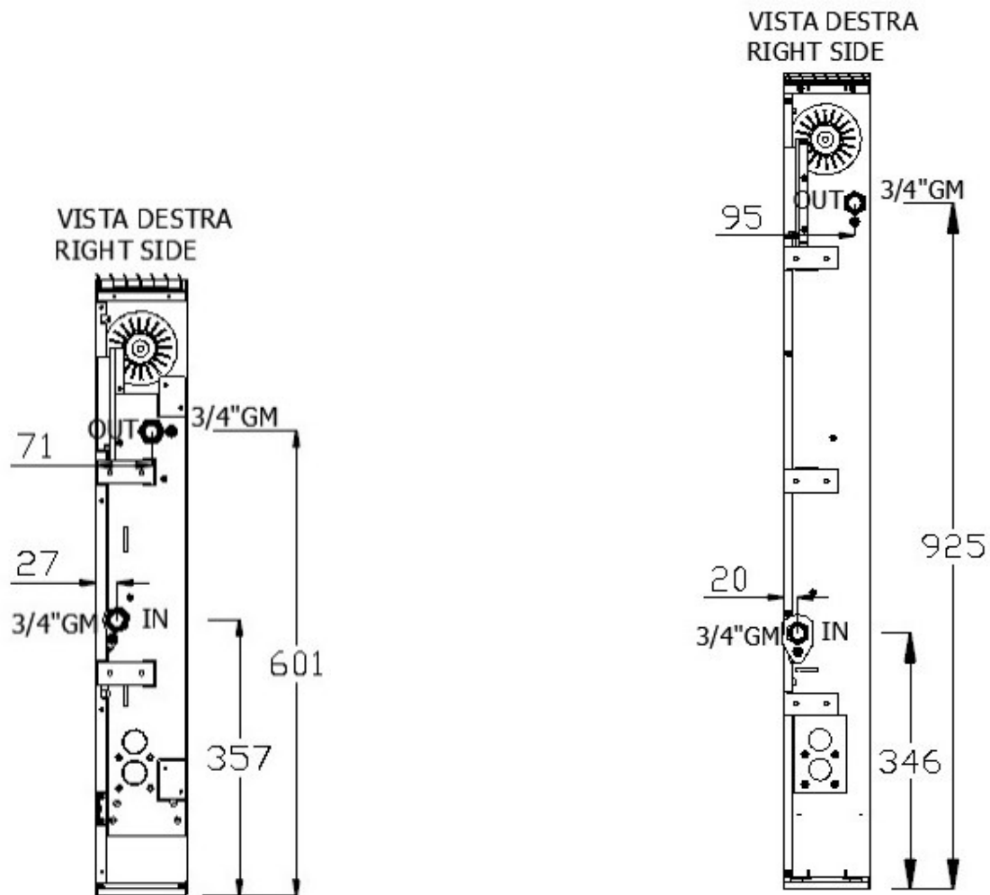
Lato destro
